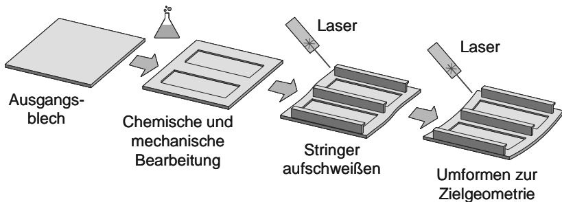
Abbildung 2: Optimierte Prozesskette in der Schalenfertigung (VÖLLNER 2004)
