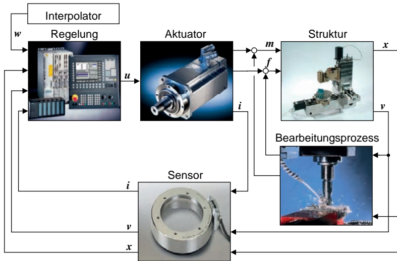
Abbildung 1-1: Die Werkzeugmaschine – ein mechatronisches Gesamtsystem
