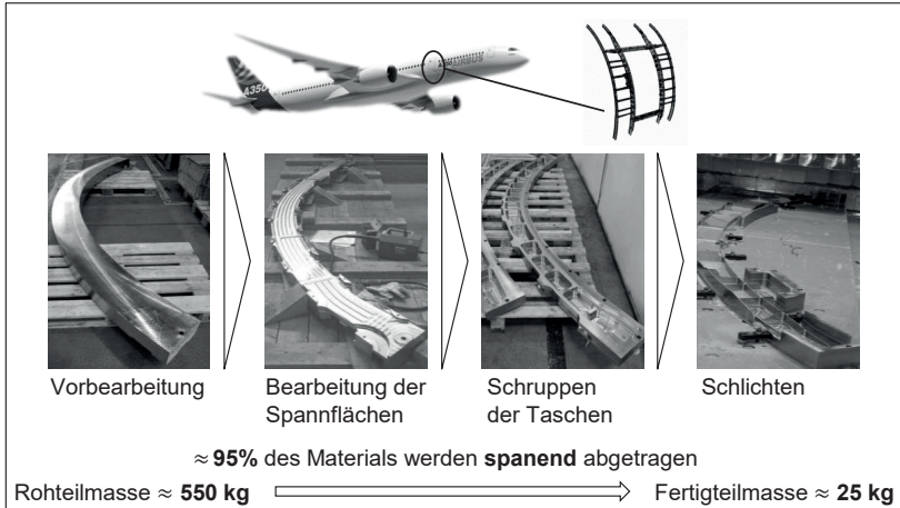
Abbildung 1-2: Spanende Bearbeitung zur Herstellung eines Luftfahrtstrukturbauteils aus Ti 6Al 4V in Anlehnung an DEGE (2015)
