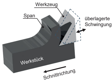
Abbildung 1-3: Prinzip der schwingungsunterstützten Zerspanung mit definierter Schneidteilgeometrie
