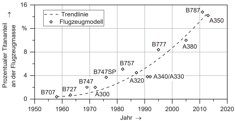
Abbildung 1-1: Prozentualer Titananteil an der Gesamtmasse bei Flugzeugmodellen der Hersteller Airbus und Boeing von 1958 (Boeing 707) bis 2015 (Airbus A350) in Anlehnung an FROES (2015)
