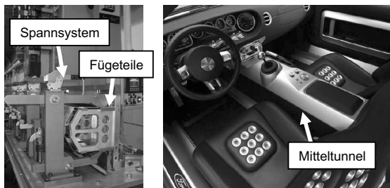
Abbildung 3: Links: Fertigung des Ford GT Mittel隧nells; rechts: Endprodukt (KALLEE 2005)
