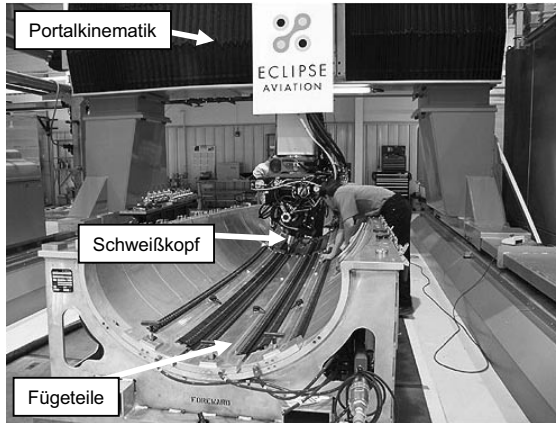
Abbildung 2: Portalkinematik zur Fertigung der Rumpfstruktur des Flugzeuges Eclipse 500 (ECLIPSE 2004)
