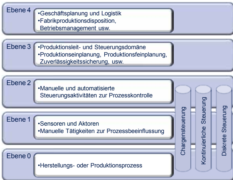
Bild 1.5: Planungsebenen nach EN 62264-1
